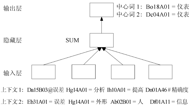
图 2 训练词义向量的神经网络结构
