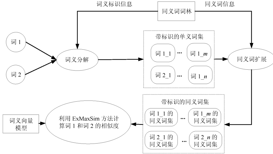
图3 基于词义向量的词语语义相似度计算过程
