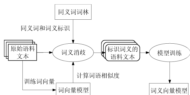
图 1 词义向量模型的构建流程
