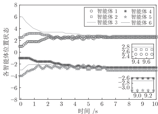
图 3 \gamma = 1, \eta = 1 智能体位置状态轨迹
