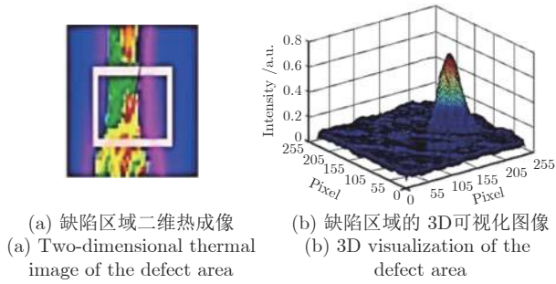
图 6 合金样品的缺陷区域热成像 3D 模型
