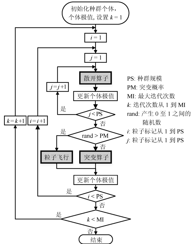
图 5 算法流程图 Fig. 5 Algorithm flowchart
