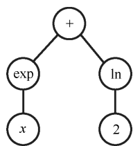
图 1 语法树
