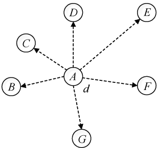
图 4 散开算子 Fig. 4 Scattering operator
