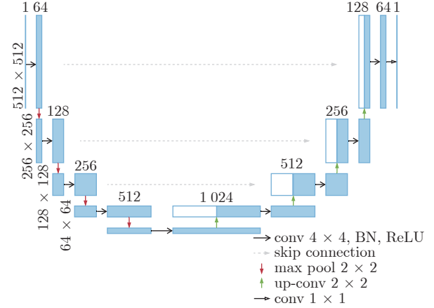
图 2 生成器网络结构
