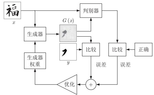
图 4 生成器训练过程
