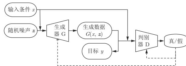
图 1 CGAN 基本框架
