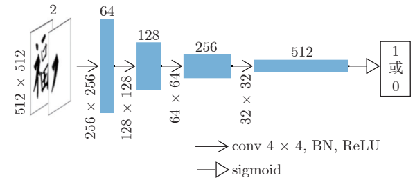
图 3 判别器网络结构
