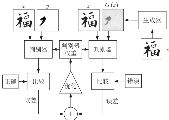
图 5 判别器训练过程
