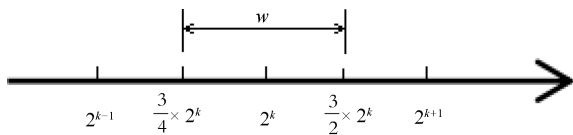
图 1 网络权值的量化规则
