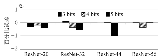
图 3 码本中无 0, SQC 和 DQC 的量化比较
