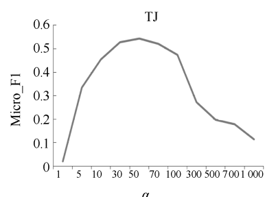
(a3) Micro_F1 值 (a3) Micro_F1 value
