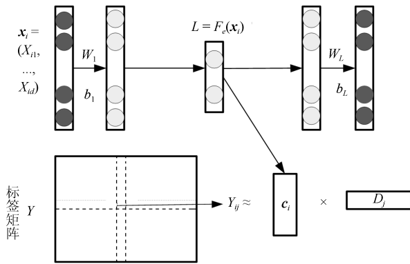
图 2 Deep AE-MF 算法模型图
