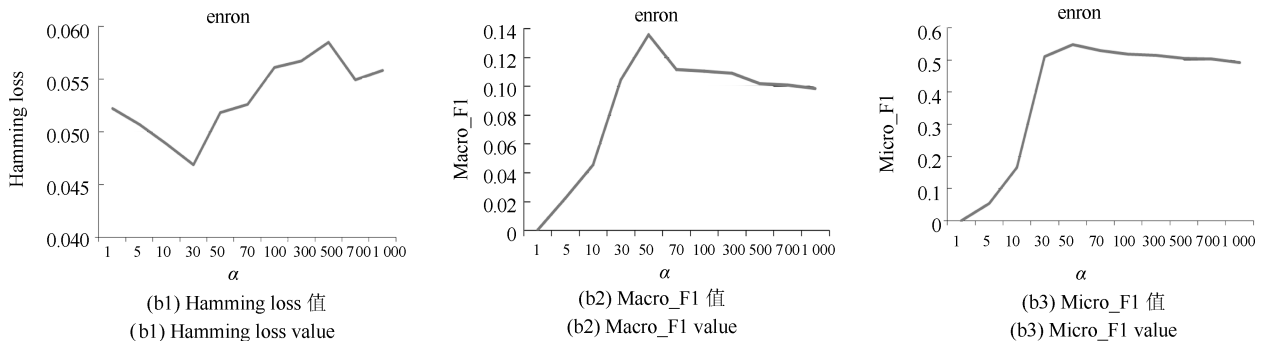
图 3 \alpha 的不同取值对数据集 TJ 和 enron 使用不同度量方式的性能体现
