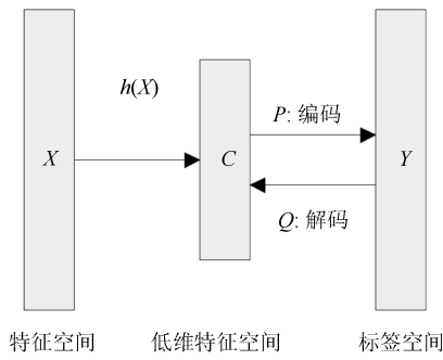
(b) 标签嵌入 (b) Label embedding
