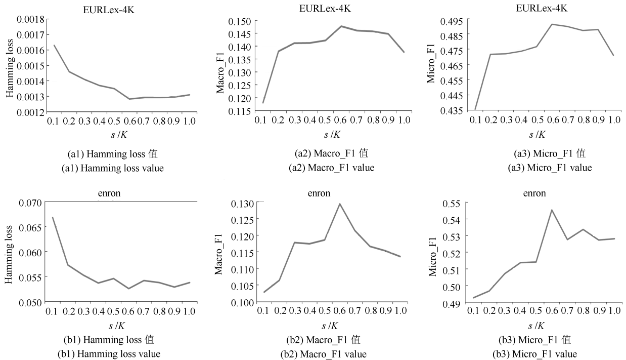
图 4 s/K 的不同取值对数据集 EURLex-4K 和 enron 使用不同度量方式的性能体现
