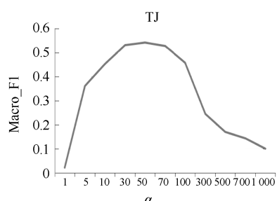
(a2) Macro_F1 值 (a2) Macro_F1 value
