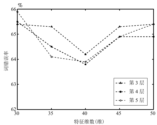
(b) Vystadial_cz 低资源识别任务 (b) Vystadial_cz low-resource task
