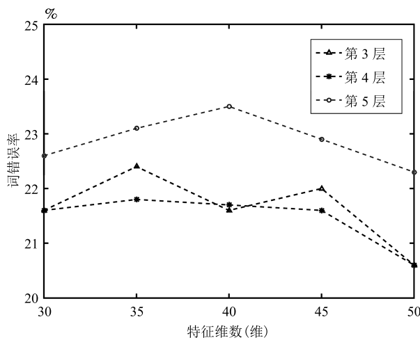
(a) Vystadial_en 低资源识别任务 (a) Vystadial_en low-resource task
