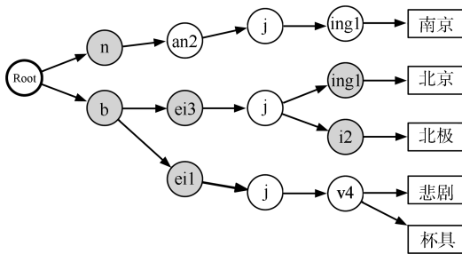
(a) 音素前缀树示例
