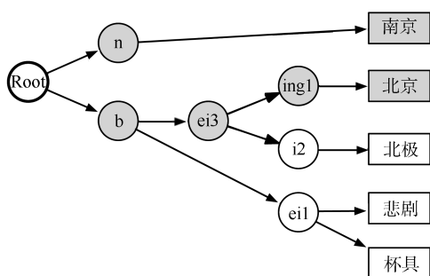
图 2 快速语言模型预测树副本生成算法 (阴影部分表示高阶语言模型历史状态特有的语言模型分数和预测分数, 即增量计算部分)
