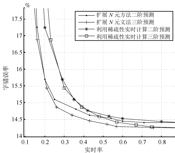
图 7 扩展 N 元文法模型方法和利用稀疏性实时计算方法的字错误率-实时率曲线
