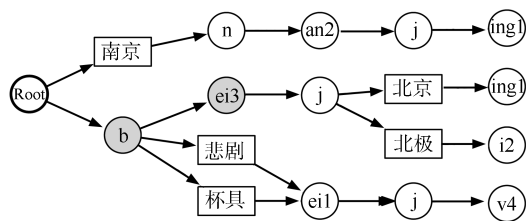
(a) 前推词尾节点后的音素前缀树
