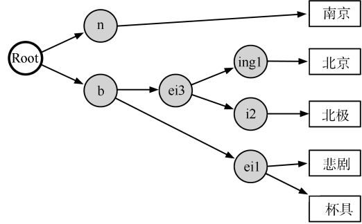
(b) 语言模型预测树示例
