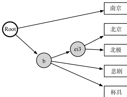
(b) 前推词尾节点后的语言模型预测树
