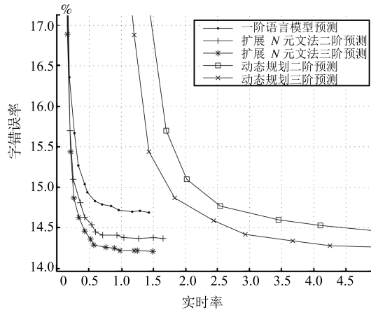
图 6 动态规划方法与扩展 N 元文法模型方法的字错误率-实时率曲线
