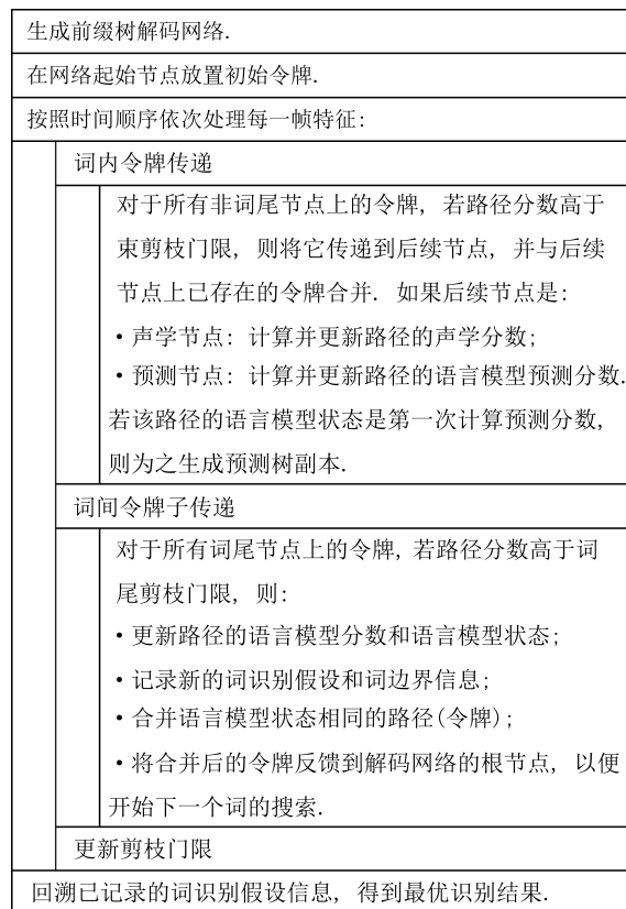
图 5 基线系统搜索算法流程图
