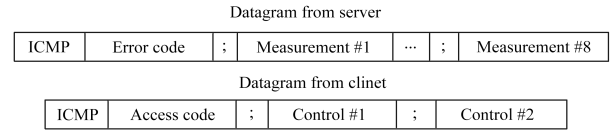
图 1 ARTT 数据包结构
