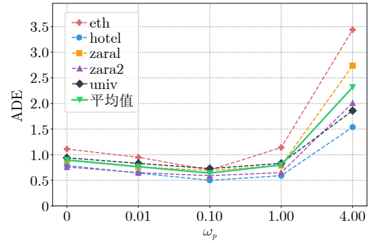
图 B1 不同 \omega_p 取值下 PI-STGCN 的 ADE 性能 Fig. B1 ADE performance of PI-STGCN with different \omega_p values
