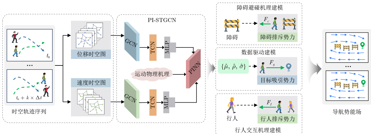
图 6 基于物理信息时空图卷积的人群移动导航势能场模型
