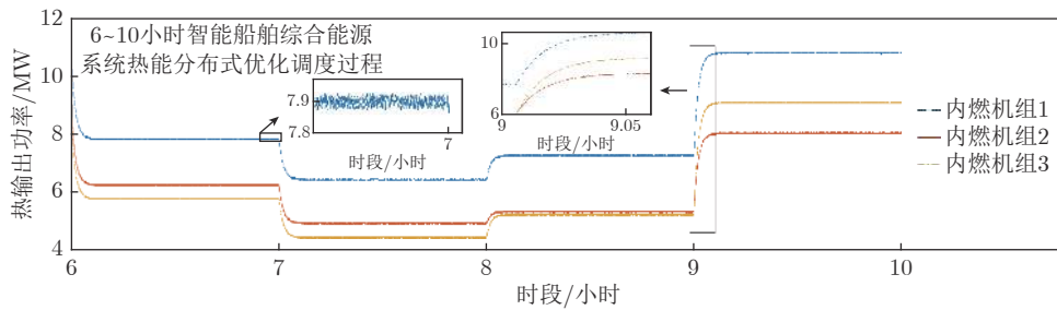
图 5 船舶航行 6~10 小时时段各供电设备热输出功率
