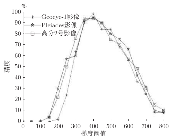
图 7 梯度阈值分析
