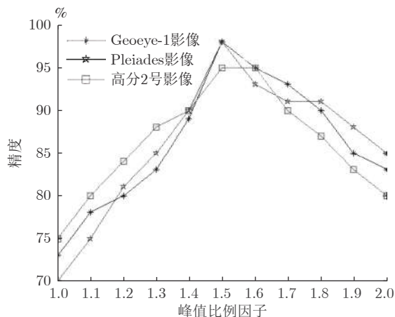
图 8 峰值比例因子分析
