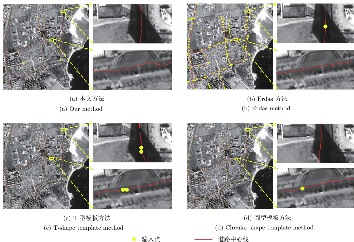
图 12 高分 2 号影像道路中心线提取
