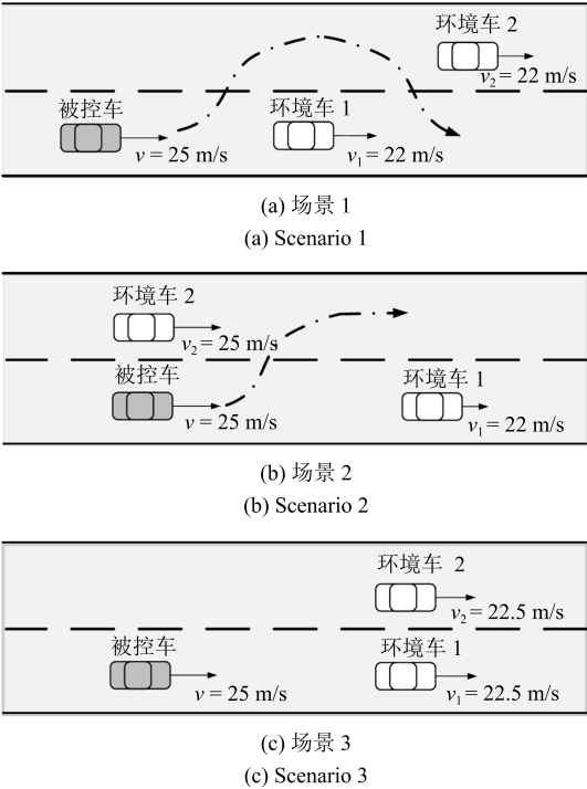
图 5 各场景示意图 Fig. 5 Sketch of each scenario
