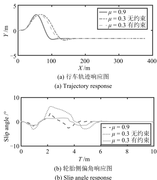
图 10 场景 4 的行车轨迹和轮胎侧偏角响应图
