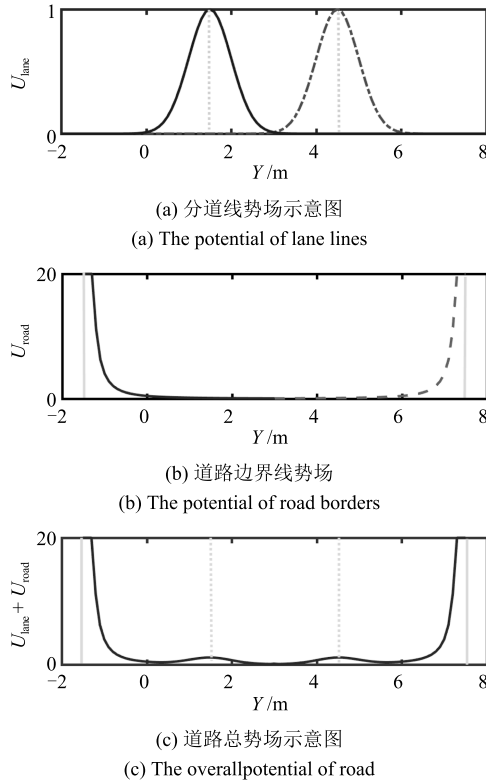
图1 道路势场示意图
