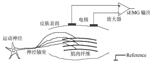
图 2 采集 sEMG 信号
