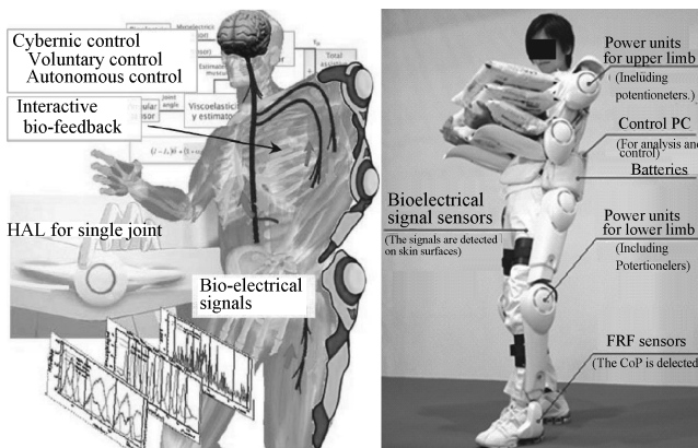
图 12 HAL 外骨骼
