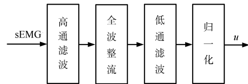
图5 一种提取肌肉活跃度 u 方法
