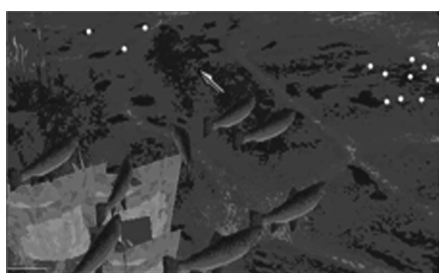
图 11 鱼群觅食
