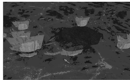
图 8 避障成功
