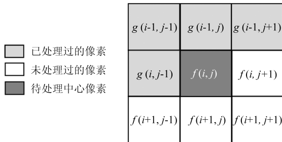
图 1 3 \times 3 的递归形式的滤波窗口
