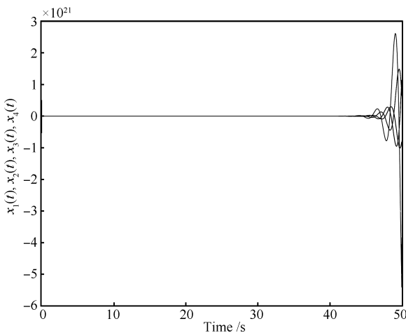
图 3 式 (24) 零输入 LTD-DD 系统的状态响应
