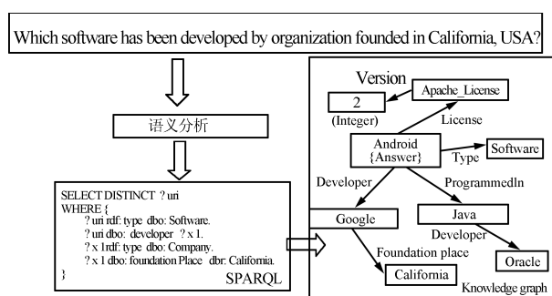
图 1 知识库问答过程
