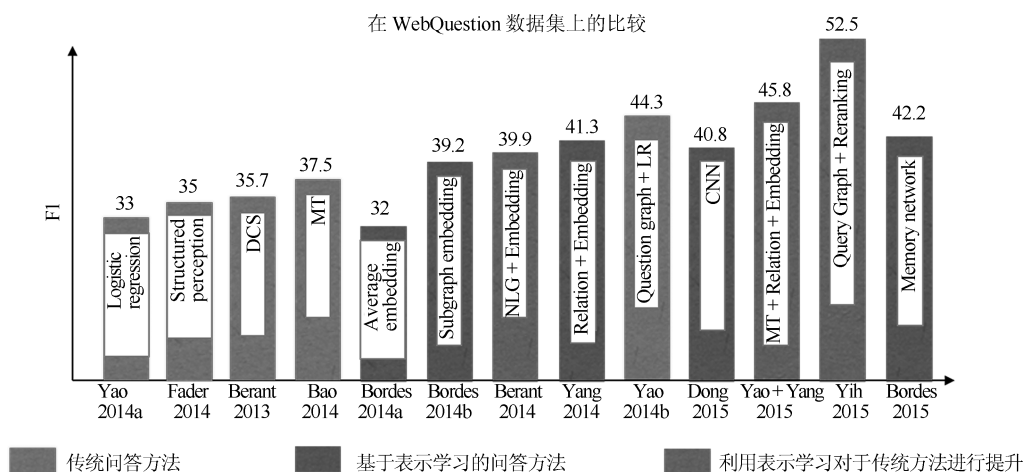
图 2 基于表示学习的知识库问答方法与传统方法的性能比较
