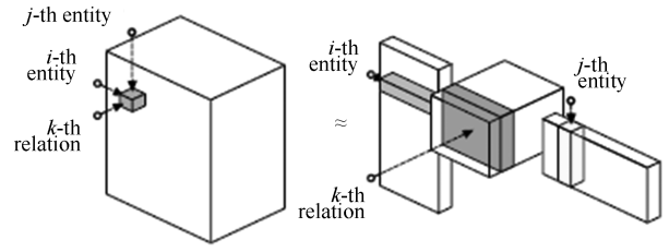
图 4 RESCAL 系统原理 [15]
